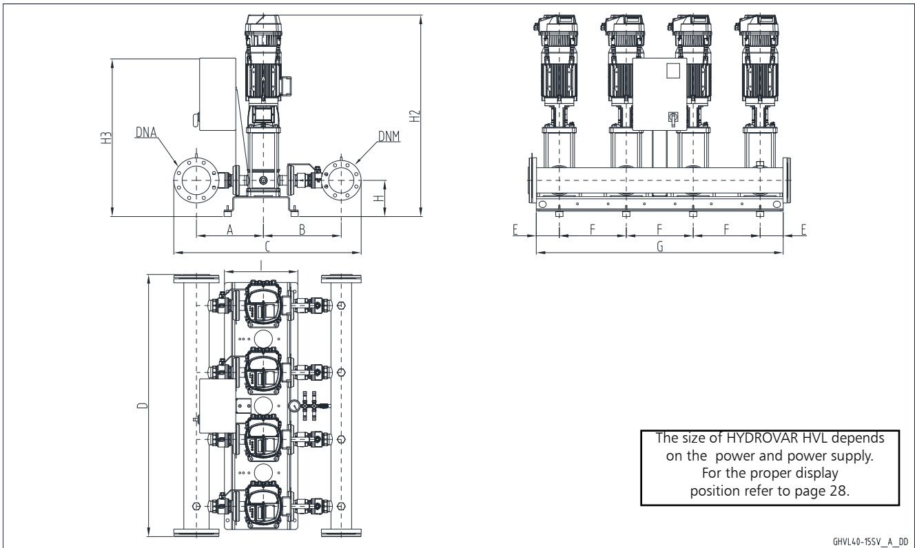
GHV40-15SV_A_DD
